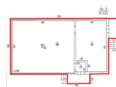
Лит. А Н= 3.33 Пит 1: Площадь, планируемая к сдаче в аренду 122.5 кв.м.
